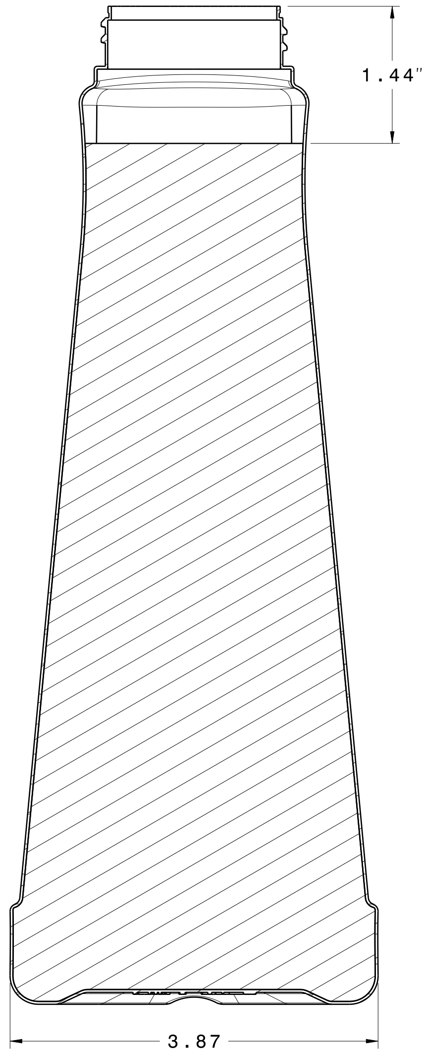
Section view A-A Scale: 1:1
