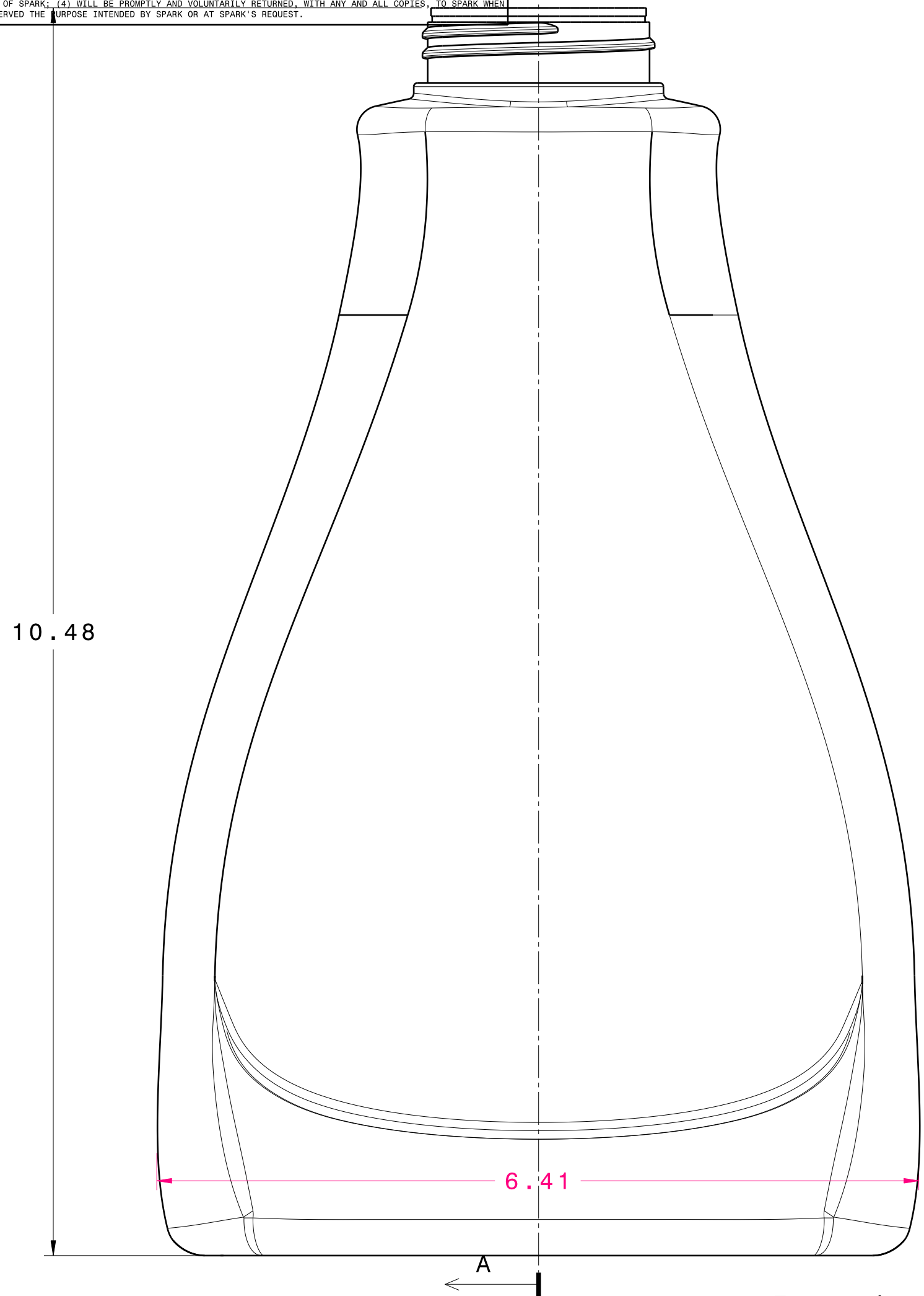
Front view Scale: 1:1
